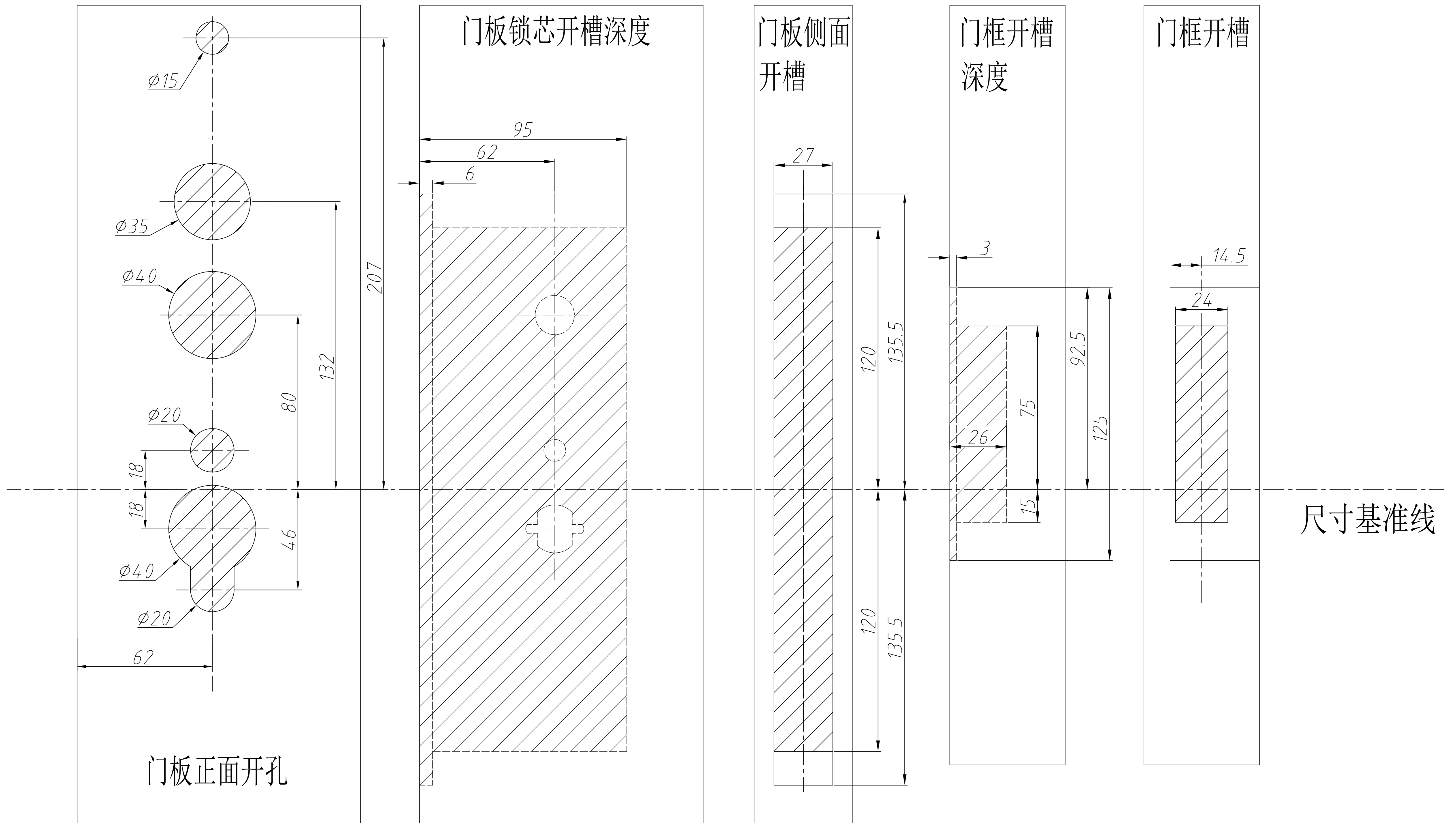
E4031配M10(方侧板)开孔图
